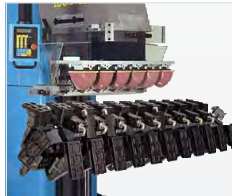
Convogliatore MEM 30°-144 su Logica 200 Conveyor MEM 30°-144 fixed on Logica 200
