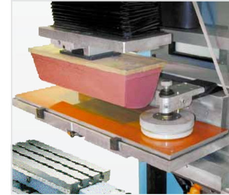
Dispositivo di ractatura a rinfresco RTE 990 e tavola ortogonale TO 201 su Logica 08 Doctoring refresher system and cross table TO 201 fixed on Logica 08
